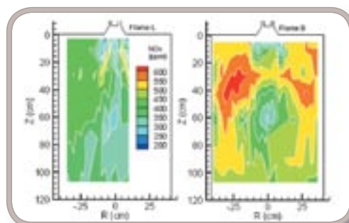
Моделирование пламени
